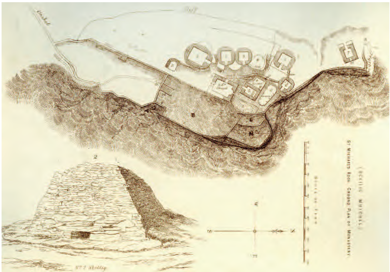
Pl. 5 An chéad phlean mionsonraithe den mhainistir ar Sceilg Mhichíl, a foilsíodh in Notes on Irish Architecture le Dunraven, iml. 1, sna 1870idí.
